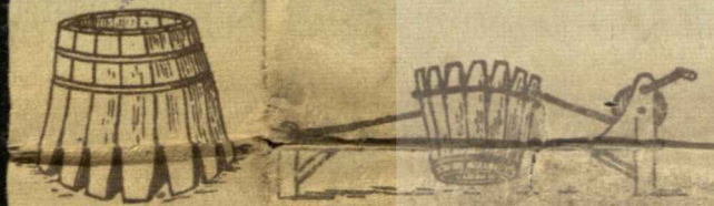
рис. 1. Остов бочки, собранный на 2 обруча. рис. 2. Стяжка остова бочки при помощи ворота.
